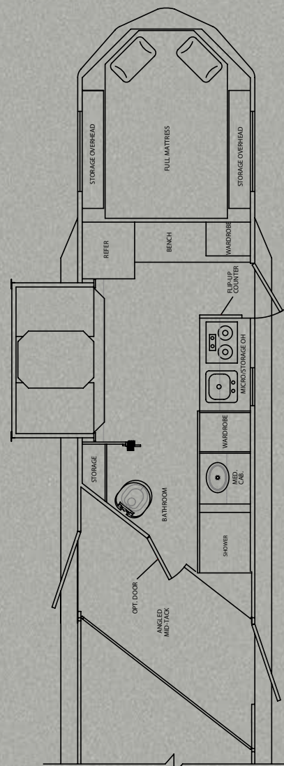
10 X 15 SLIDE OUT AMT
